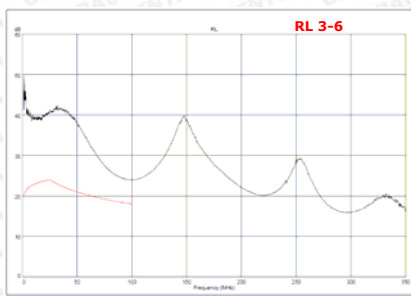
Τυπικές μετρήσεις Patch Cord CAT5E μήκους 1 μέτρου
