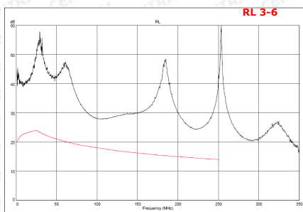
Τυπικές μετρήσεις Patch Cord CAT 6 μήκους 1 μέτρου
