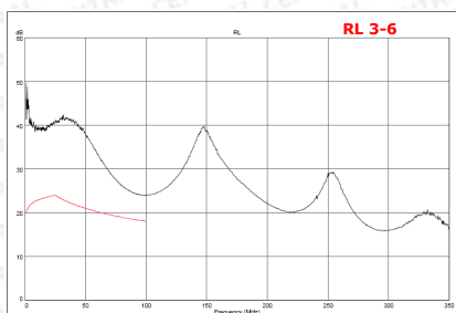
Τυπικές μετρήσεις Patch Cord CAT5E μήκους 1 μέτρου
